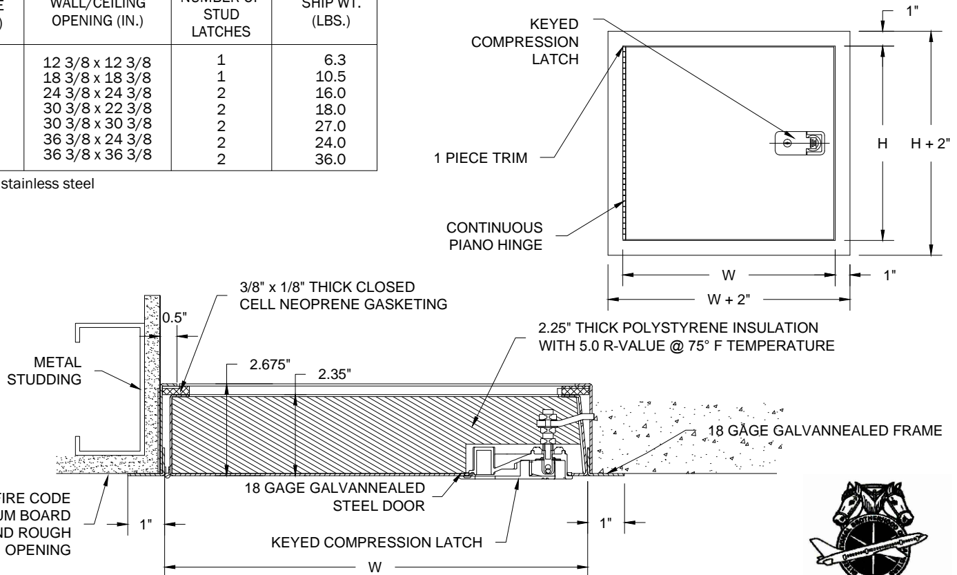
SECTION A-A
